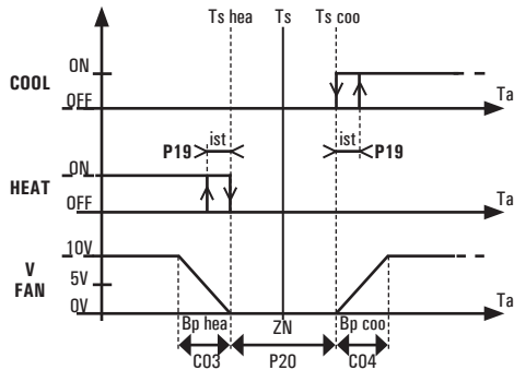
Fig. 15: Le schéma montre le pilotage des vannes dans un système à 4 tuyaux avec zone neutre. De façon analogue, la sortie de la vanne chaude (HEAT) d'un système à 2 tuyaux sera pilotée de la même manière ; dans ce cas-là, la T_s (température du point de consigne) coïncidera avec la T_s hea en hiver et avec la T_s coo en été. Le schéma ne tient pas compte de l'action éventuelle du temps d'intégration et présume que la sortie proportionnelle du ventilateur (V FAN) est configurée pour action directe ( P05=0 ) et pour un signal 0-10 V ( C15=0 ; C16=100 ). La sortie proportionnelle du ventilateur est toujours éteinte (0 V) quand la sortie de la vanne (COOL ou HEAT) est éteinte (ce cas n'est pas visible sur le schéma).
