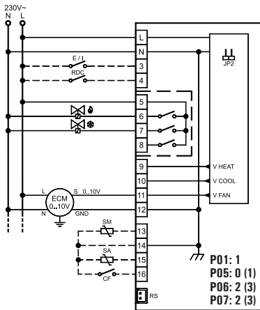
Fig. 8: Schéma de connexion pour pilotage de deux actuateurs on/off à 230V ~ pour installation à 4 tubes et pilotage proportionnel du ventilateur. Esquema de conexión para el pilotaje de dos actuadores on/off a 230V ~ para instalación a 4 tubos y pilotaje proporcional del ventilador.
