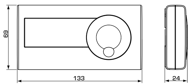
Установочные размеры для комнатного модуля
