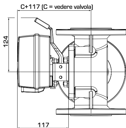
Dimensioni di installazione dell'unità di controllo serie CRA120
