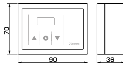
Dimensioni di installazione della casetta di controllo
