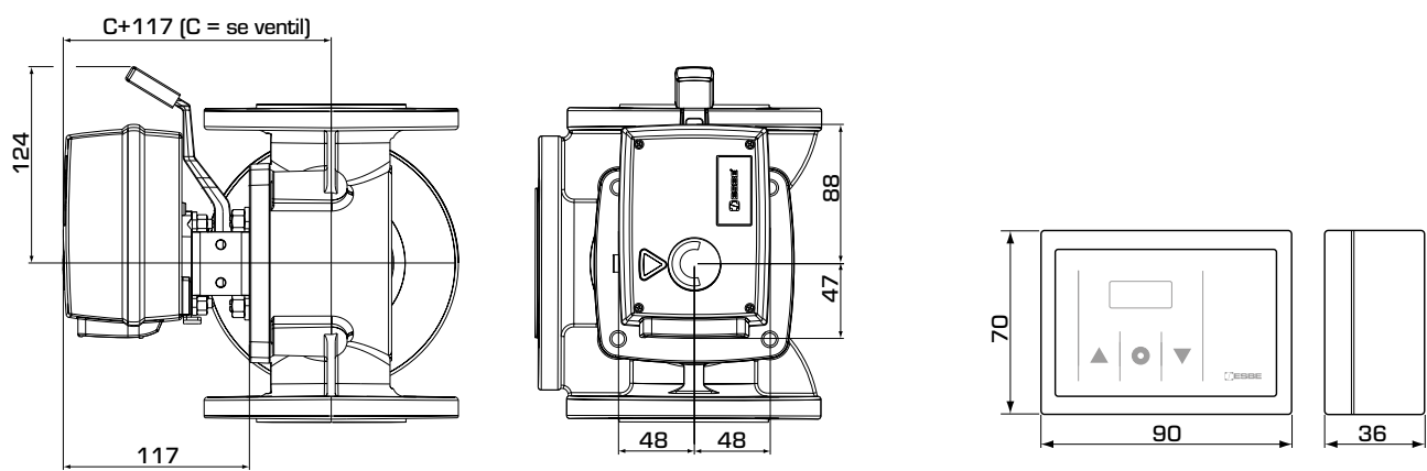
Installationsmått för reglering, serie CRA120
