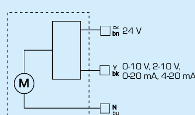
Ställdon serie ARA659
