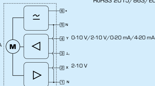
Ställdon serie ARA639
