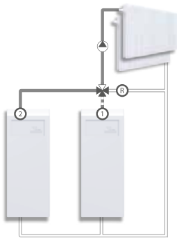
Fuentes de calor en paralelo
