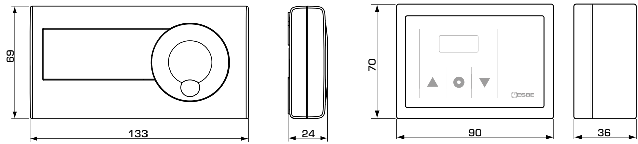
Dimensioni di installazione della cassetta di controllo
