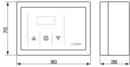
Dimensiones de instalación para la caja de control
