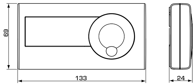
Dimensiones de instalación para la pantalla del ambiente interior
