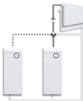
Fonti di calore in parallelo
