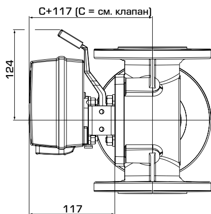
Установочные размеры для контроллеров серии CRC120
