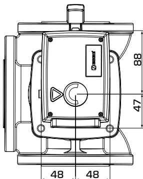
Установочные размеры для контроллеров серии CRC120
