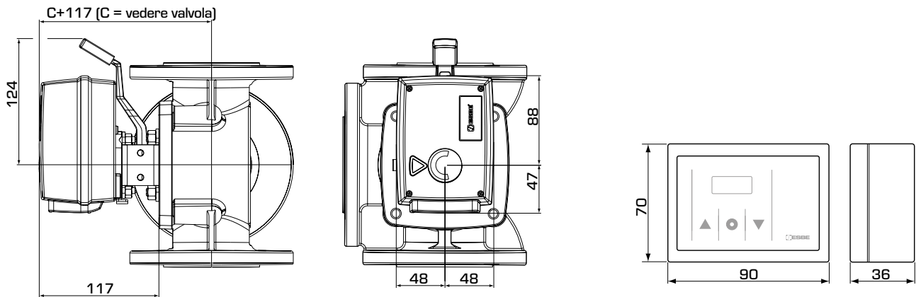
Dimensioni di installazione per l'attuatore serie CRC120 con miscelatore ESBE serie MG, G, F, T/TM, H/HG e BIV.
