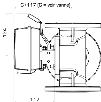
Dimensions d'installation pour les servomoteurs de la série CRC120 avec vannes de mélange ESBE des séries MG, G, F, T/TM, H/HG et BIV
