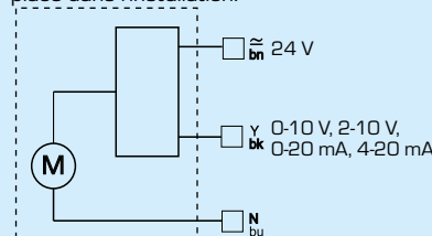
Servomoteur série ARA659
